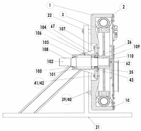
COUPE A-A
